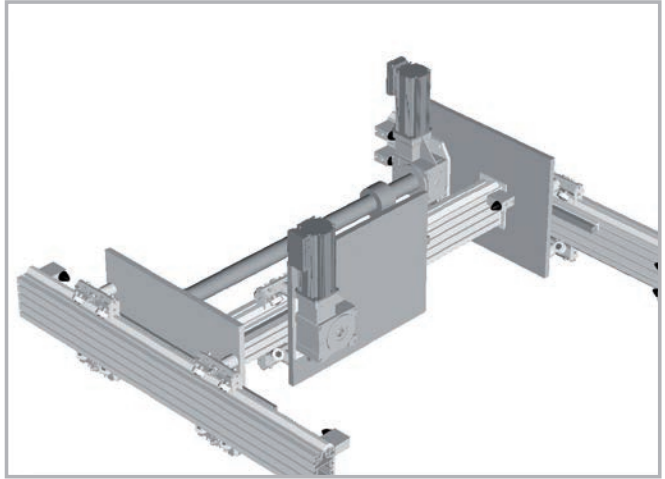
2 - Sistema Y-X de dos ejes
