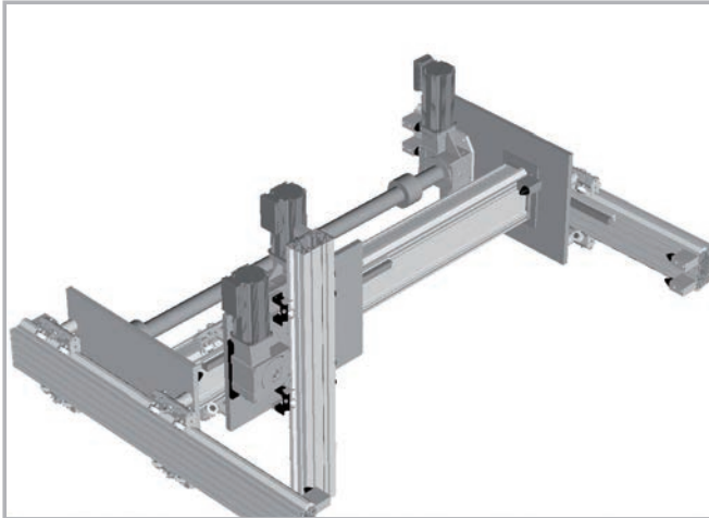
3 - Sistema de tres ejes X-Y-Z
